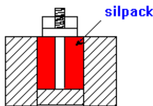
ANCLAJE DE PERNOS O VARILLAS
